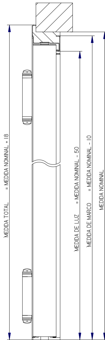
CORTE A-A 1:6
