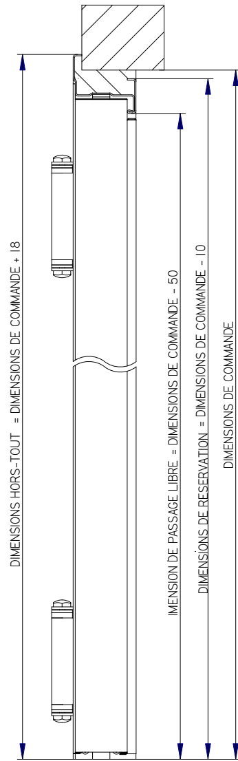
VUE EN COUPE A-A 1:6
